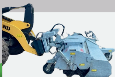
Balayeuse hydraulique
